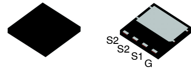
PQFN4 8X8 2P CASE 483AP
