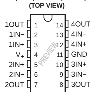
TLV344 . . . D (SOIC) OR PW (TSSOP) PACKAGE
