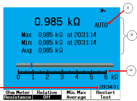
Figura 2 Pantalla del Multímetro
