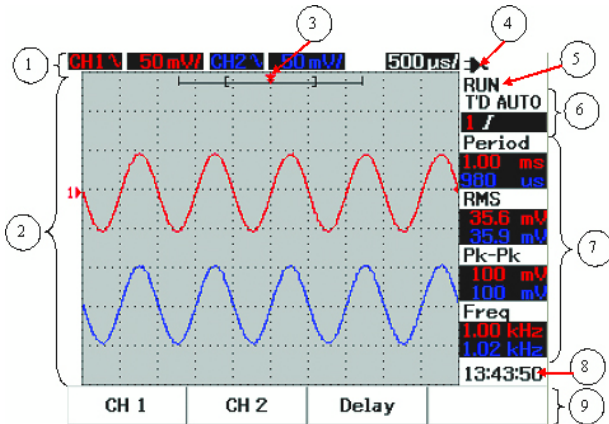
Abbildung 1 Oszilloskopanzeige
