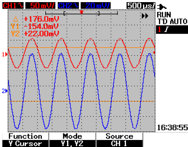
Abbildung 5 Cursor-Messanzeige
