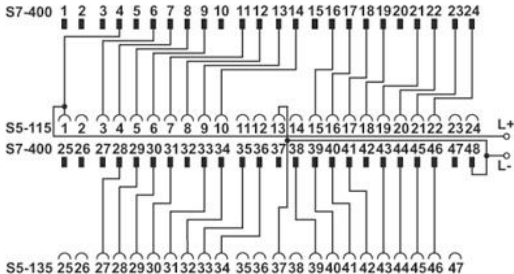
FLKM S115-465-7LA/UI/S400 connection scheme
