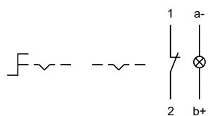
Wiring diagram 15
