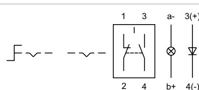
Wiring diagram 20
