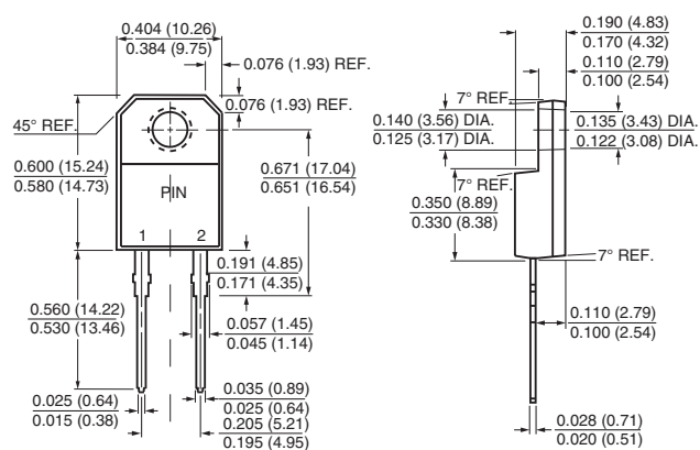
ITO-220AC
