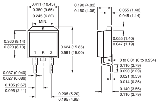
D 2 PAK (TO-263AB)
