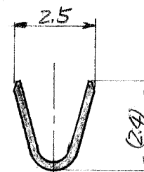
断面 A-A
