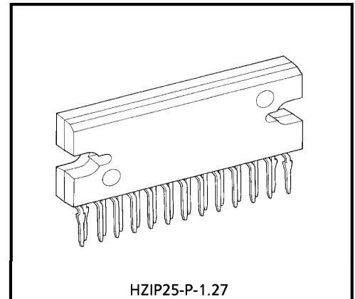
HZIP25-P-1.27
