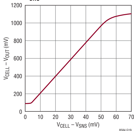
V_{SNS} Transfer Function
