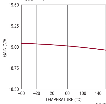
V_{SNS} Amplifier Gain
