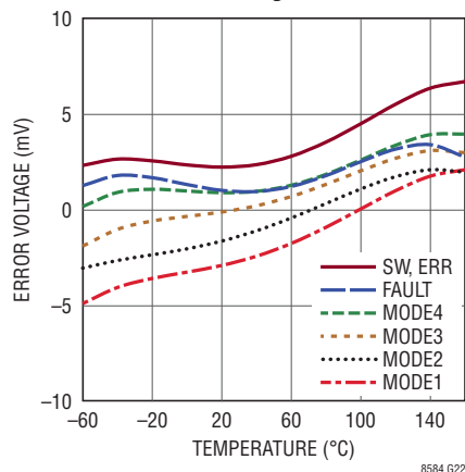
Handshake Voltage Error
