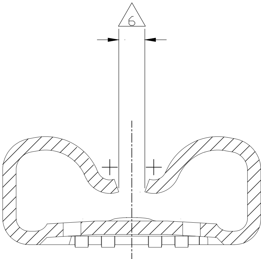
SECTION A-A
