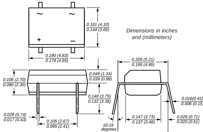
Case Style MBM
