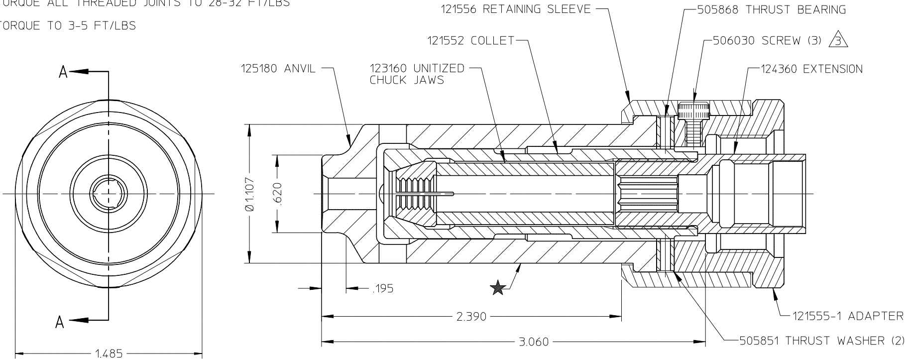
SECTION A-A
