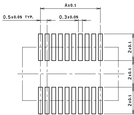
参考基板レイアウト MOUNTING LAYOUT
