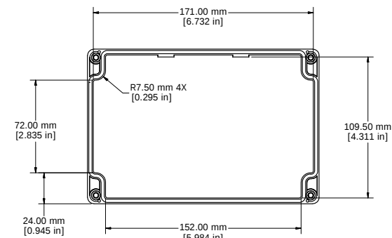
LID - INSIDE
