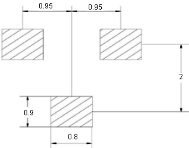
Dimensions : Millimetres
