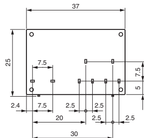
2 \text{ CO}
