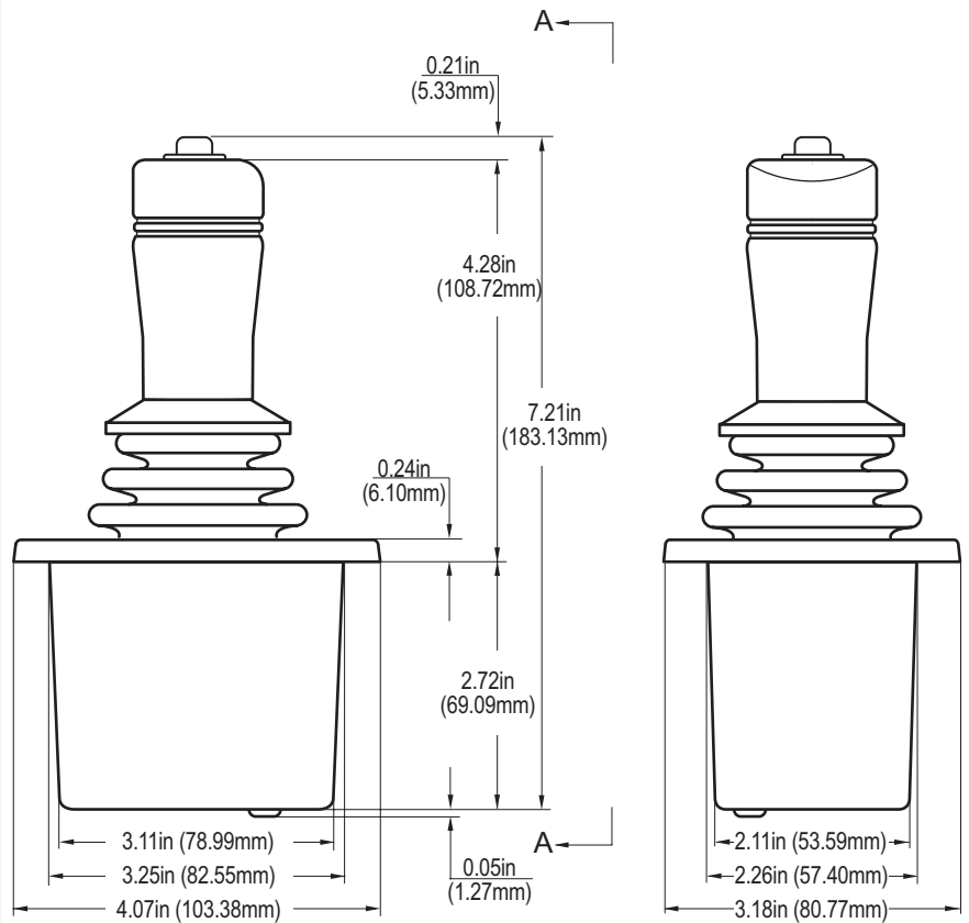
VIEW A-A
