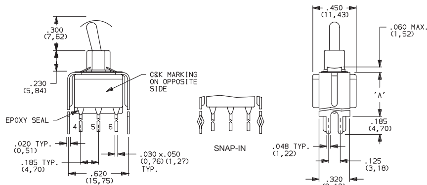
E201MD1_BE DPDT
