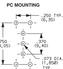
E101MD1_BE SPDT
