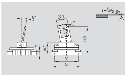
Flexible actuator AZ 335/355-B6-Flex
