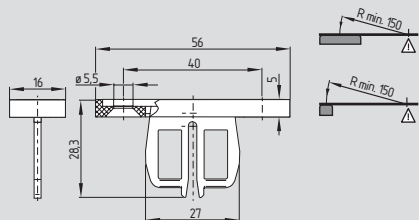
Straight actuator AZ 15/16-B1
