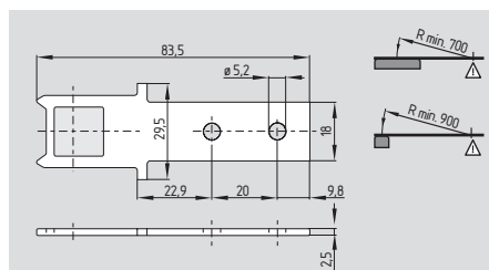
Straight actuator AZ 335/355-B1
