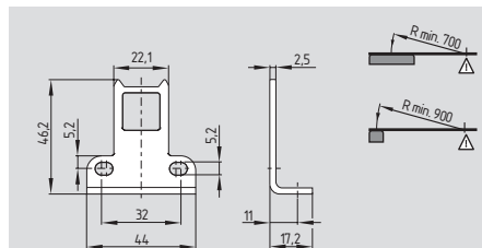
Angled actuator AZ 335/355-B5
