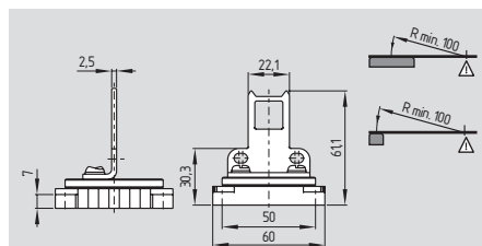
Angled actuator AZ 335/355-B5-Flex
