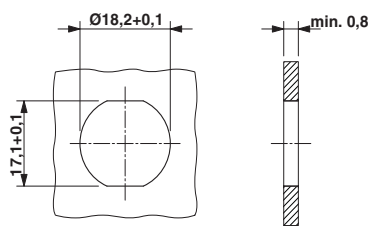
Einbaumaße: ST-17.1N8A6100S, Bohrung mit Verdrehsschutz und Kontermutter (Empfehlung bei Einbau in Stahlblechwand)
