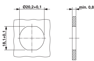
Einbaumaße: ST-17.1N8AH100S, Bohrung mit Verdrehsschutz und Kontermutter (Empfehlung bei Einbau in Stahlblechwand)
