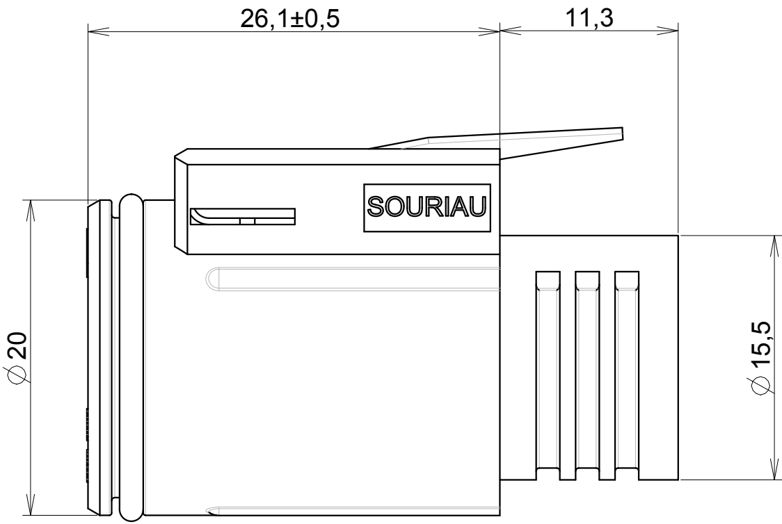
ECHELLE 3/1
