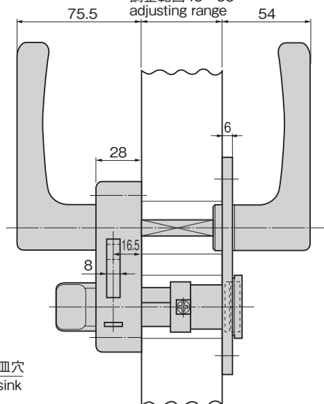
パネル厚 Panel thickness 調整範囲45~55 adjusting range
