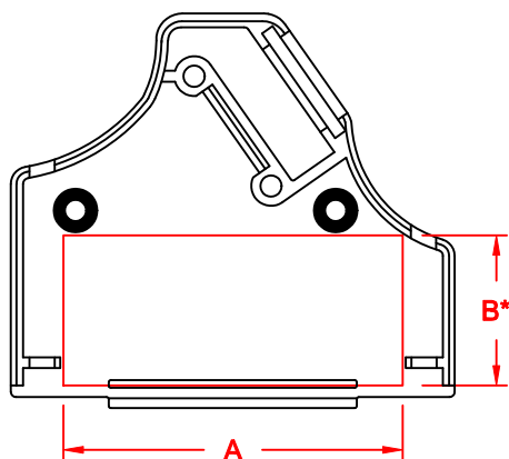
25-PIN
