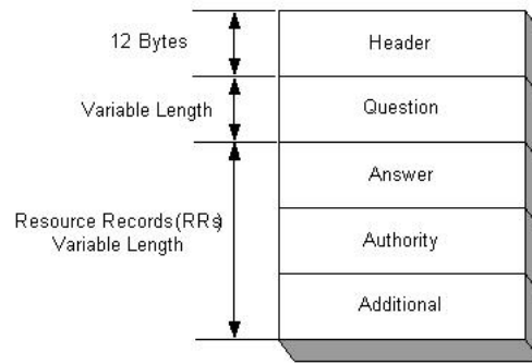
<Fig 3.34: DNS Message Format>
