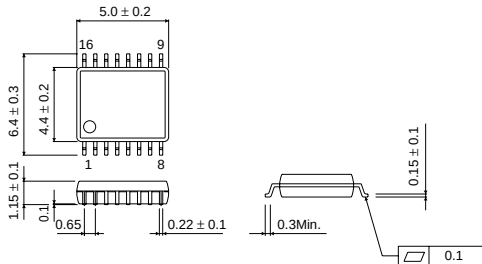
SSOP-B16
