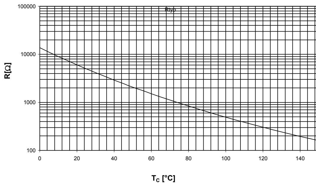
NTC- Temperaturkennlinie (typisch) NTC- temperature characteristic (typical)
