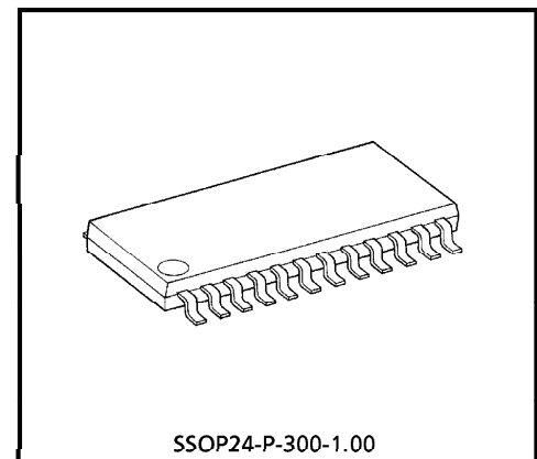
SSOP24-P-300-1.00 Weight : 0.32g (Typ.)
