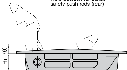
パネル穴明け寸法 Panel drilling dimensions (FA-816-1, FA816-2)
