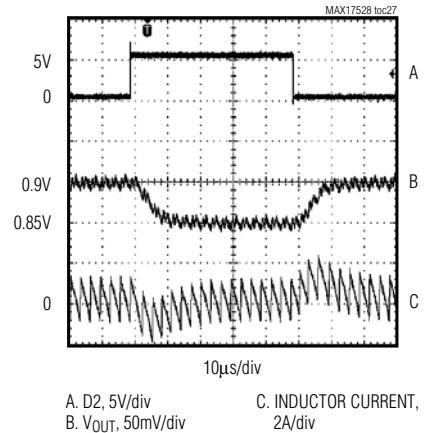
D2 50mV DYNAMIC VID CODE CHANGE
