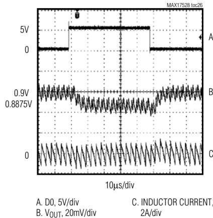
D0 12.5mV DYNAMIC VID CODE CHANGE
