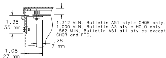
DETAIL Y
