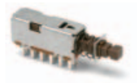
PN41LGSA02QE 4PDT
