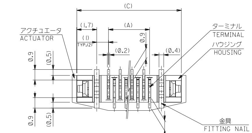
下面図 BOTTOM VIEW
