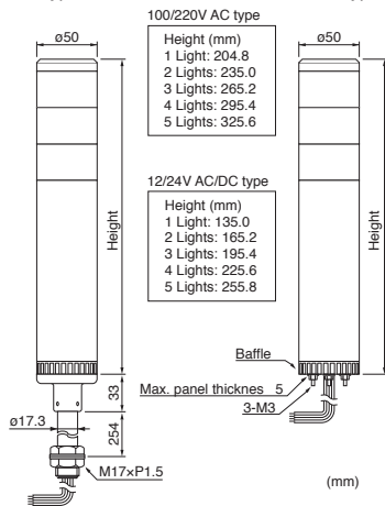
LE type
