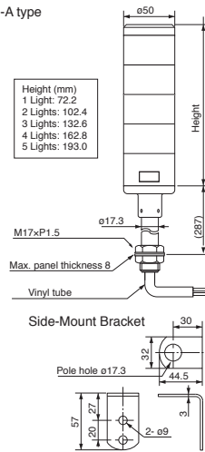
LES-A type
