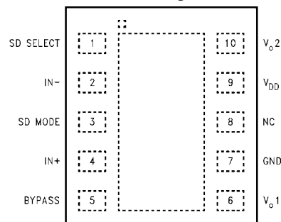
LLP Package
