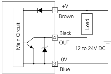
NPN Output
