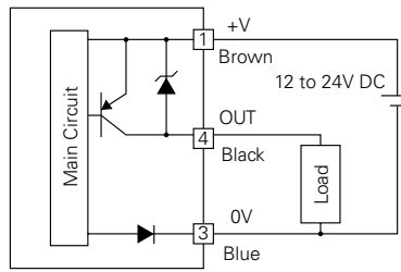
PNP Output
