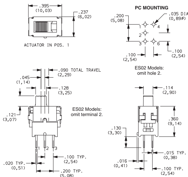
ES01MCBE SPDT
