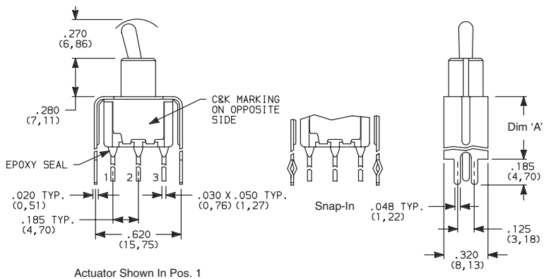
7101MD9__BE SPDT
