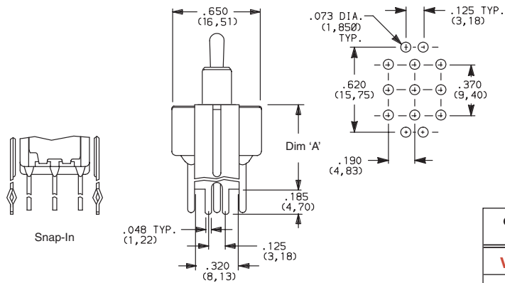
7301MD9__BE 3PDT
