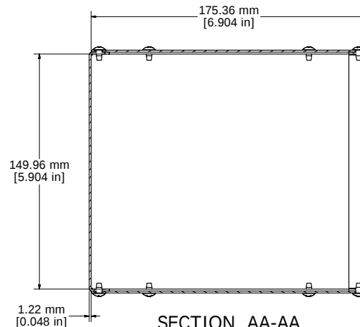
SECTION AA-AA
