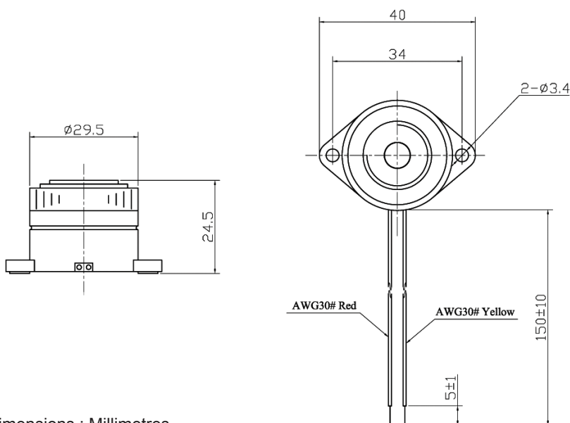
Dimensions : Millimetres
