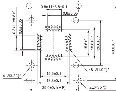
IC51-0484-081 (48 Pins)
