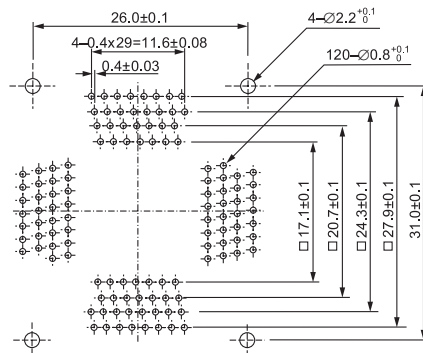
IC51-1204-1812 (120 Pins)
