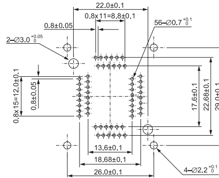
IC51-0564-924 (56 Pins)
