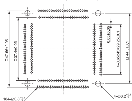
IC51-1844-1541 (184 Pins)
