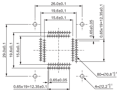
IC51-0804-956-2 (80 Pins)
