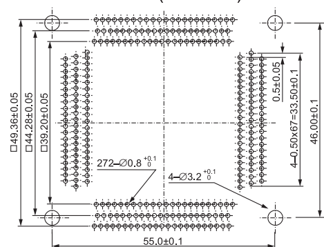
IC51-3044-1471-2 (304 Pins)
