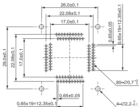
IC51-0804-795 (80 Pins)
