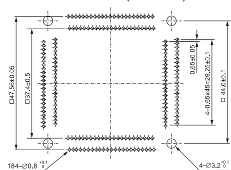
IC51-1844-1148-1 (184 Pins)
