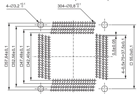
IC51-3044-1471-5 (304 Pins)
