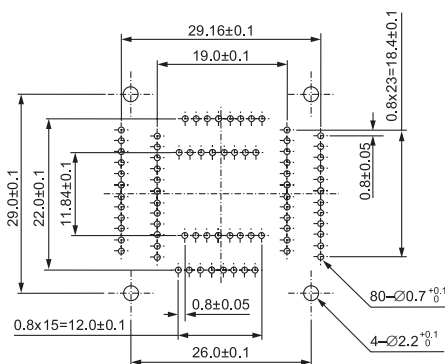
IC51-819-KS12720 (80 Pins)
