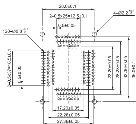
IC51-1284-844-1 (128 Pins)
