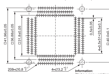
IC51-2084-1052-* 2 (208 Pins)
