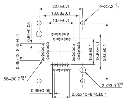
IC51-0564-680 (56 Pins)
