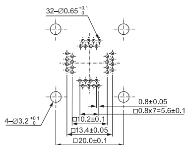
IC51-0324-354 (32 Pins)
