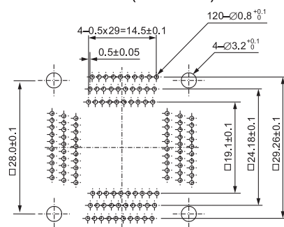
IC51-1204-1652 (120 Pins)
