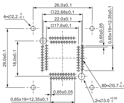
IC51-0804-956-2 (80 Pins)
