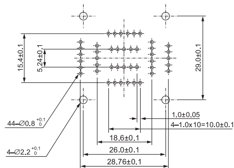
IC51-0444-615 (44 Pins)
