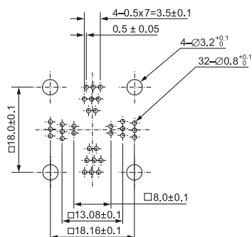
IC51-0324-805 (32 Pins)
