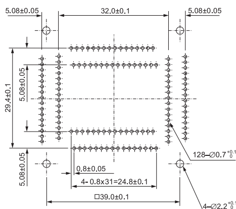
IC51-844-KS13329 (128 Pins)
