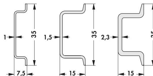
Beispiele von Tragschienenvarianten passend für KL 35
