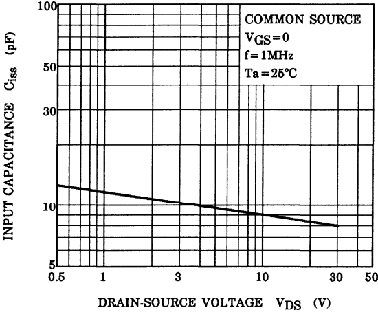
C_{iss} - V_{DS}
