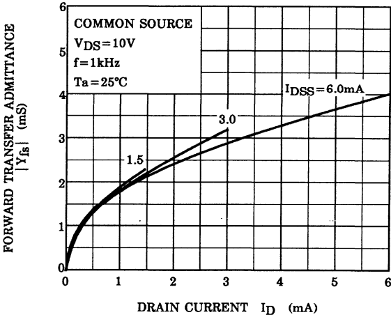
|Y_{fs}| - I_D
