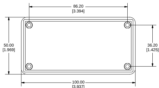
BOTTOM OF LID
