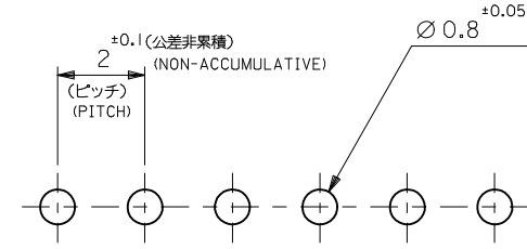
基板取付穴推奨寸法
