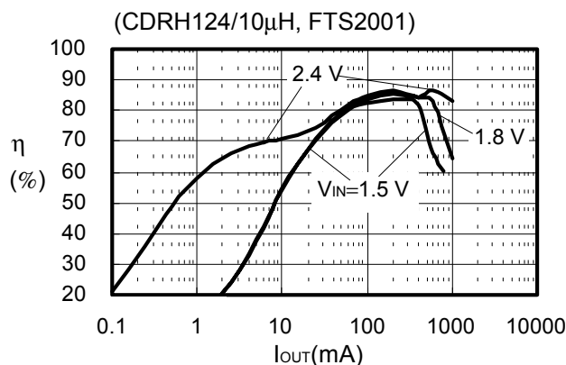
(4) S-8341A25AFT
