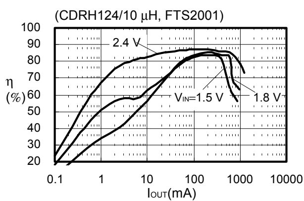
(6) S-8340A33AFT
