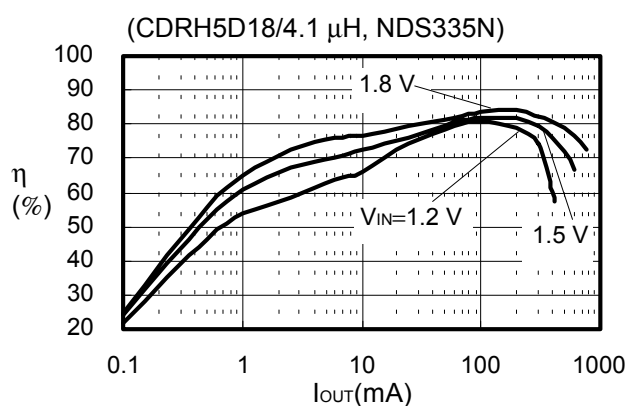
(5) S-8340A33AFT
