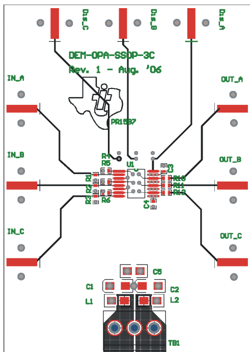
(a) DEM-OPA-SSOP-3C Top Layer
