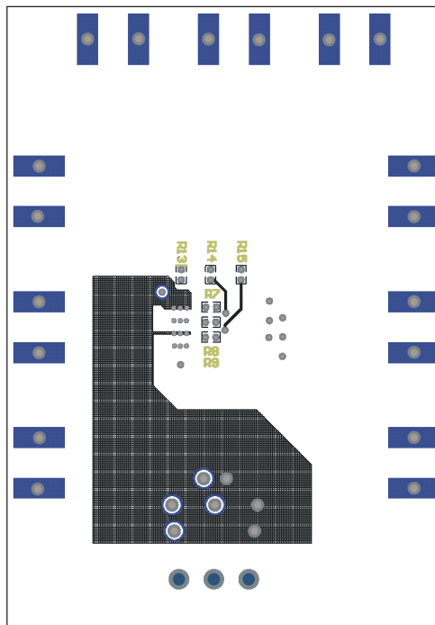
(d) DEM-OPA-SSOP-3C Bottom Layer (negative image shown for clarity)
