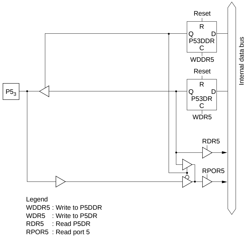
Figure C-5 (d) Port 5 Block Diagram (Pin P5 3 )
