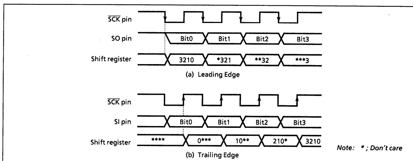
Figure 2-37. Shift Edge
