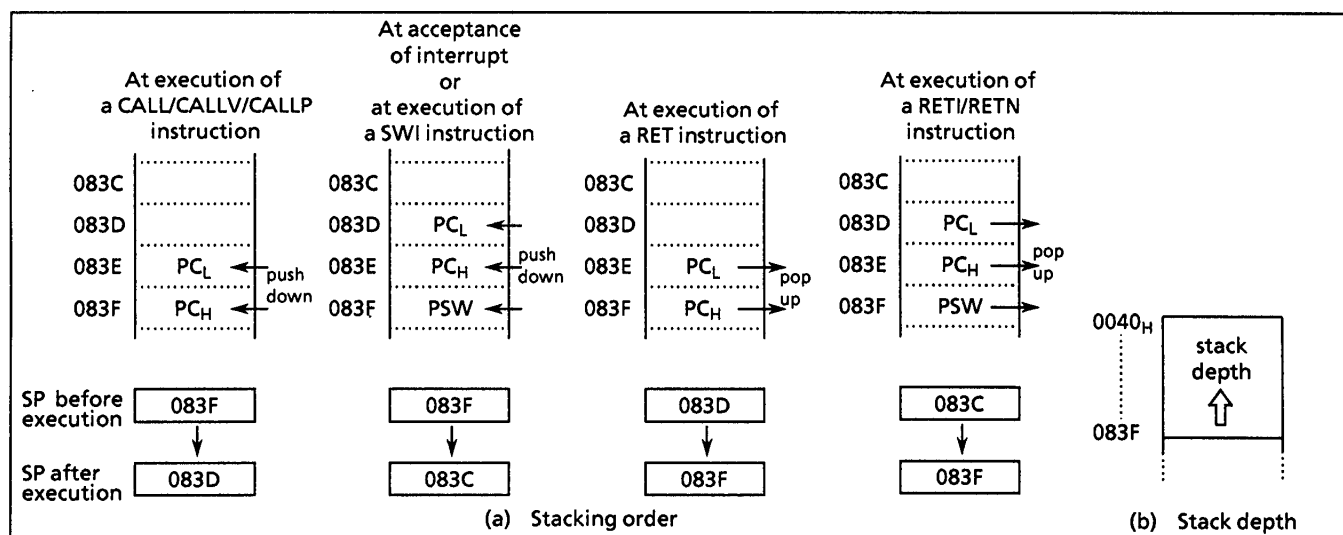
Figure 1-8. Stack
