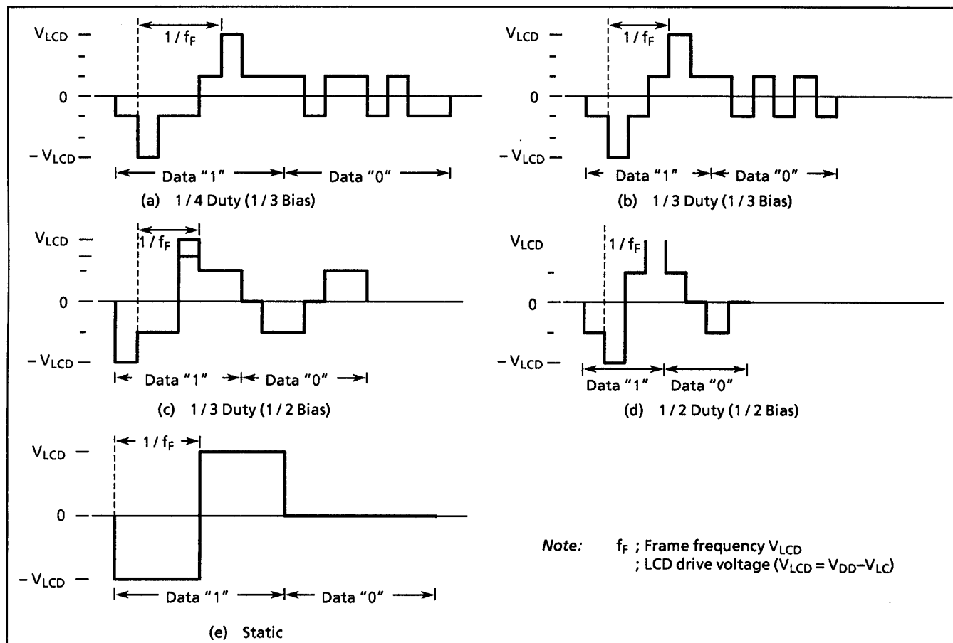
Figure 2-47. LCD drive waveform (COM - SEG pins)
