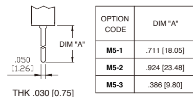
M5 Wire Wrap
