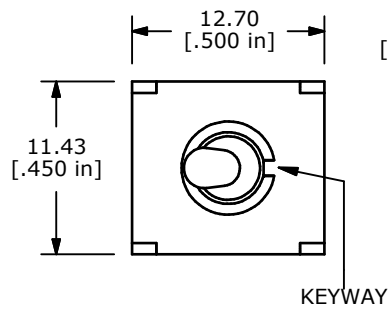
KEYWAY
